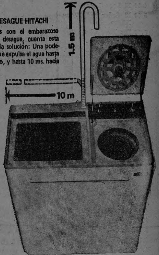
LAVADORA HITACHI MODELO PS-310P
